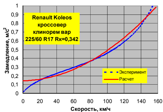
Кроссовер Renault Koleos с клиноремным вариатором (АР № 21, 2008)
