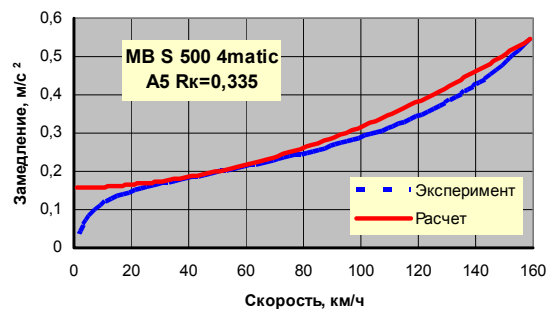
Полноприводный седан Mercedes-Benz S 500 4matic КП А5 (АР № 11, 2007)
