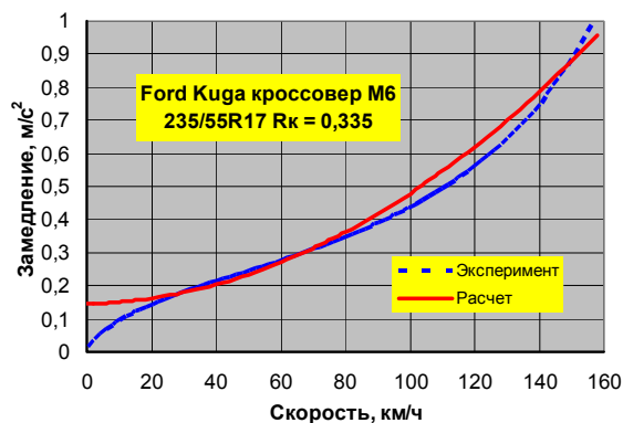
Кроссовер Ford Kuga КП М6 (АР № 21, 2008)
