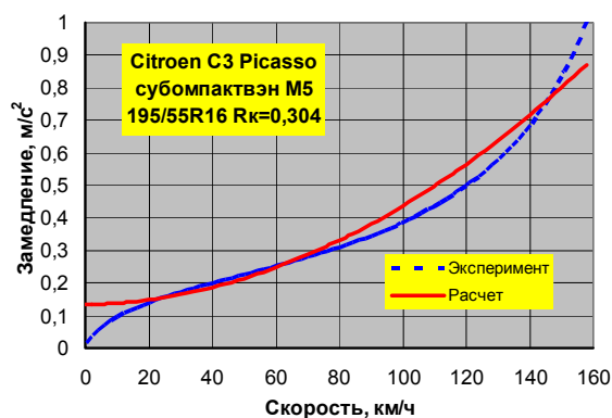
Переднеприводный субкомпактвэн Citroen C3 Picasso КП М5 (АР № 15, 2009)
