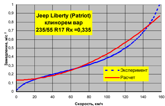
Кроссовер Jeep Liberty (Patriot) с клиноремным вариатором (АР № 20, 2007)
