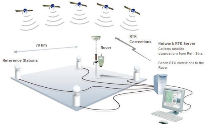
Рисунок 2 – Схема роботи в RTK режимі
