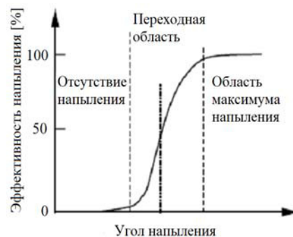
Рис. 11. Общая схема зависимости относительной эффективности напыления от угла напыления [26]
