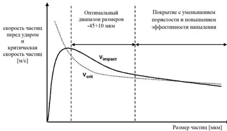
Рис. 6. Критическая скорость напыляемых частиц — v_{\text{crit}} и скорость напыляемых частиц перед ударом о подложку — v_{\text{impact}} в зависимости от размера частиц. Оптимальное распределение размеров частиц для ХГН [23]
