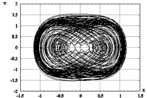
Рис. 1. Фазовый портрет системы
