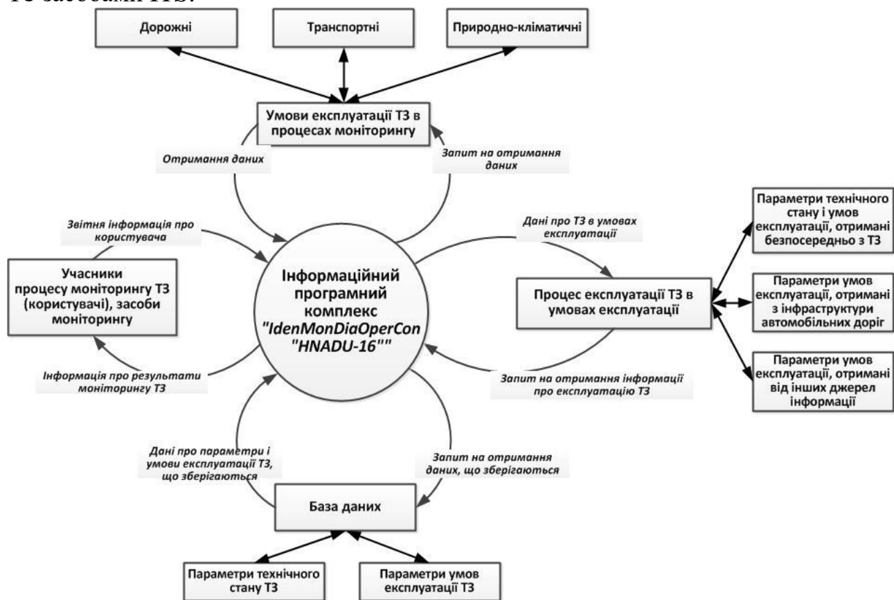
Рис. 1. DFD-діаграма функціонування інформаційної системи моніторингу ТЗ
